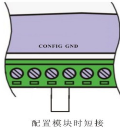
图3 ISOAD16 模块进入配置状态接线图
