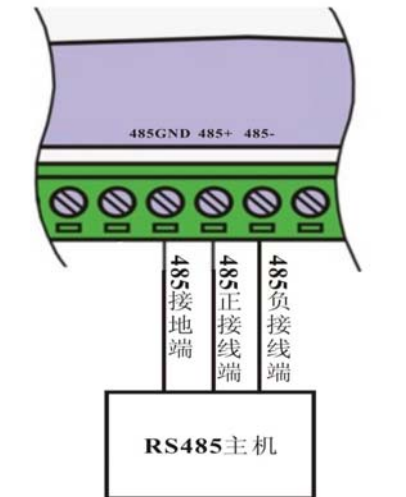
图5 ISOAD16 模块 RS-485 接口接线图
