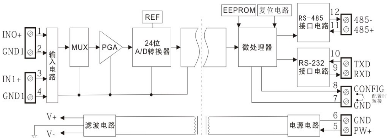
图1. ISO 4021 产品原理框图
