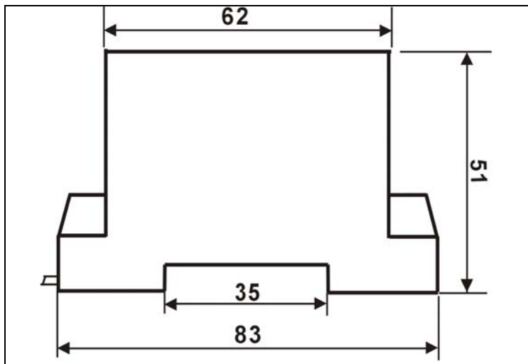
图 4. 产品正视图
